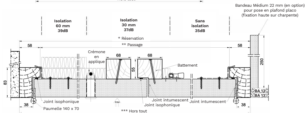
2 vantaux
