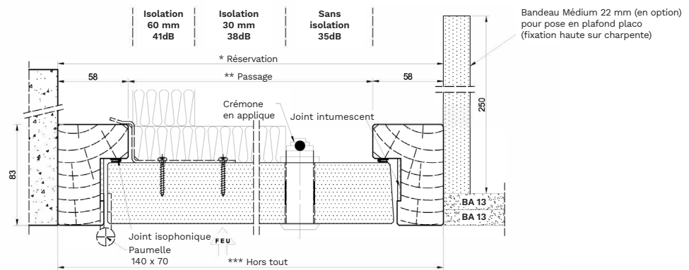
1 vantail
